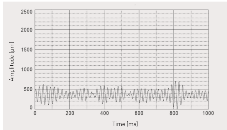
Weg-Zeit-Diagramm
